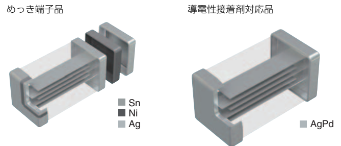
図2 積層チップサーミスタの内部構造
