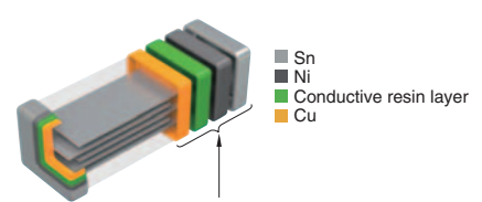
樹脂電極品
