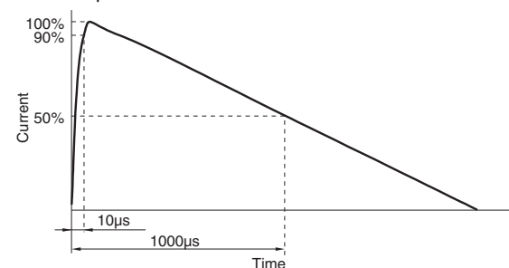
*2 10/1000µs 試験波形
