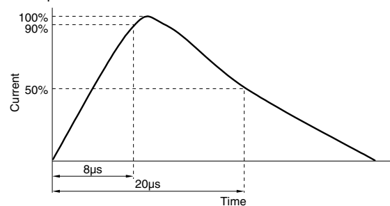
*1 8/20µs 試験波形
