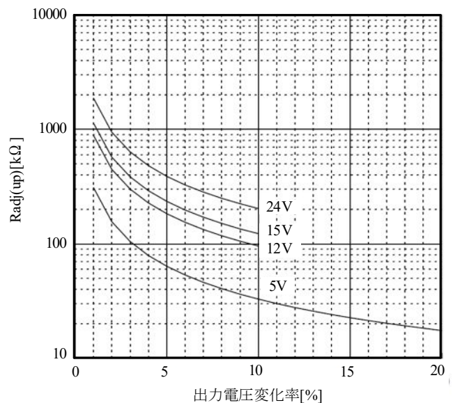
図 2-4 \Delta(\%) 對外付け抵抗(2)
