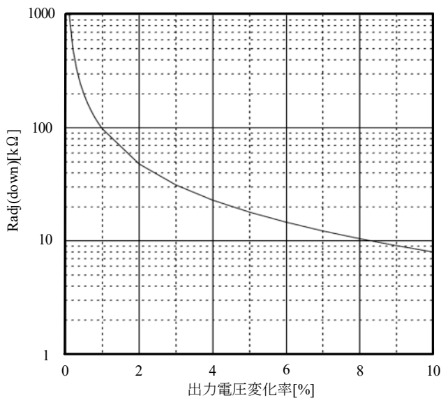
図 2-2 \Delta(\%) 對外付け抵抗(1)
