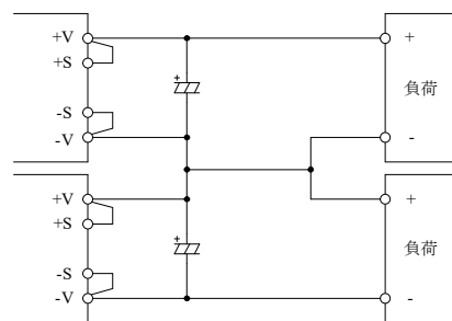
図 14-2 土出力使用の直列運転
