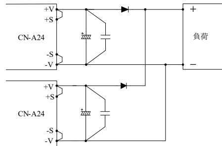
図 12-1 冗長運転接続方法
