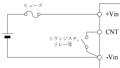
図 11-1 CNT 接続例 (1)
