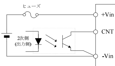
図 11-2 CNT 接続例 (2)
