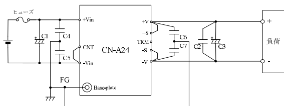
図 20-4 外付け部品接続例
