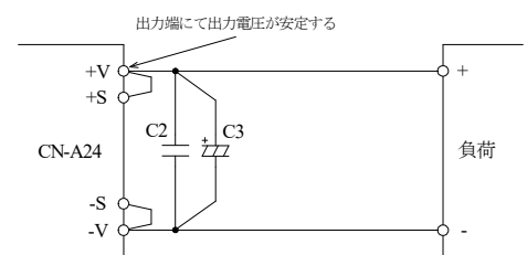
図 10-1 リモートセンシングする場合
