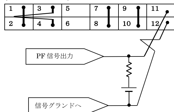
(12-60V モデル)
