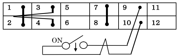
(12-60V モデル)
