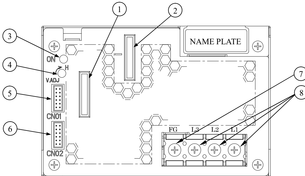
HWS1800T フロントパネル面
