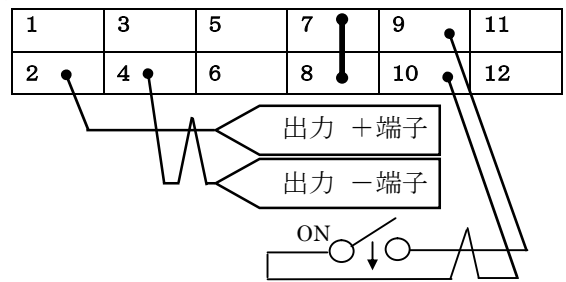
(12-60V モデル)
