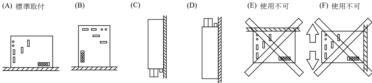
HWS1800T 3V出力ディレーティング
