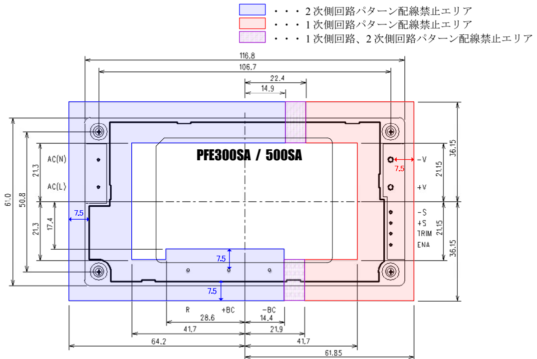
図 7-4 電源実装基板パターン配線禁止エリア（1次側回路-2次側回路間距離 7.5mm の場合）
