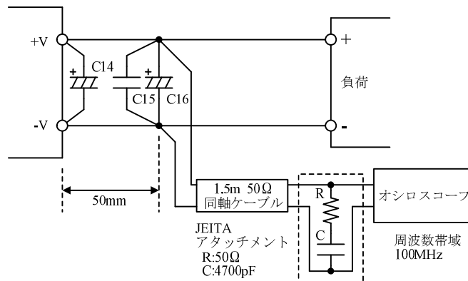
図 6-4 出力リップル電圧 (スパイクノイズ含む) 測定方法
