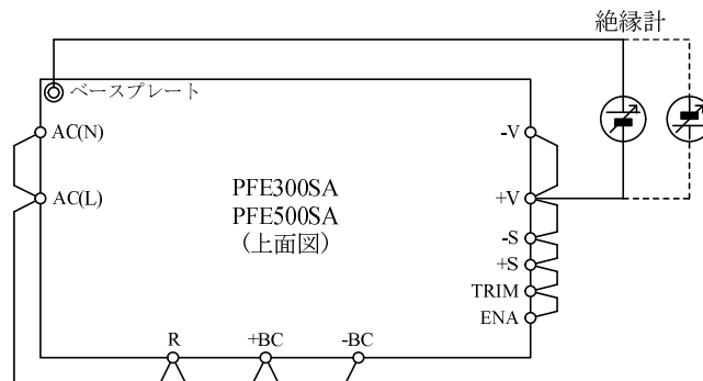
図 6-7 絶縁抵抗試験方法
