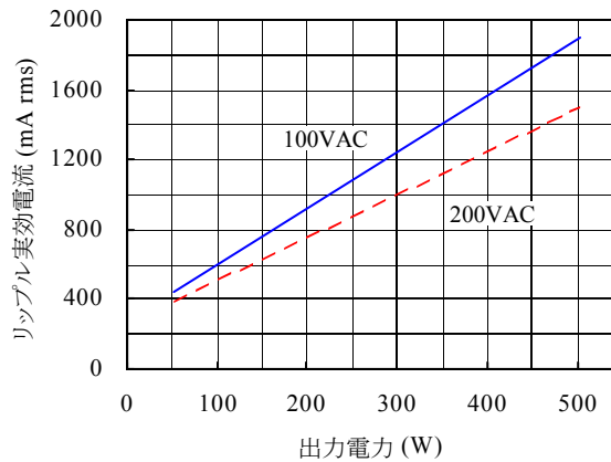
図 5-2 許容リップル電流値
