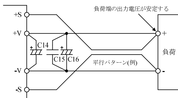
図 6-2 リモートセンシングする場合
