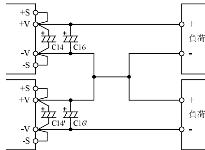
図 6-6 土出力使用の直列運転
