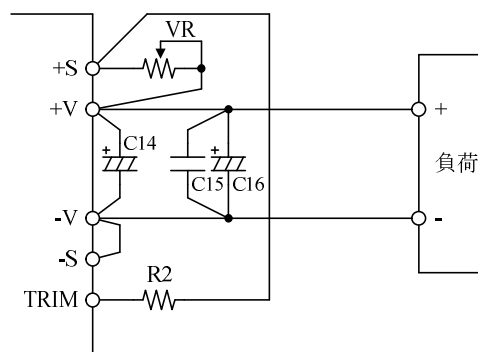
図 6-1 外付け抵抗の接続例
