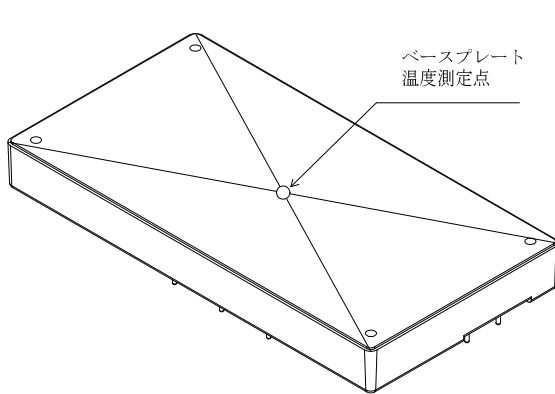
図 7-1 ベースプレート温度測定点
