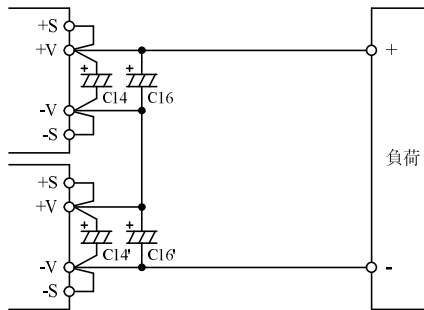
図 6-5 出力電圧積み重ね直列運転
