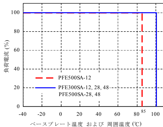
図 7-3 ディレーティングカーブ
