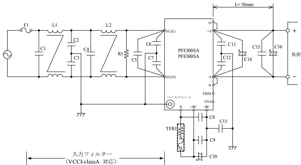
図 5-1 基本的な接続
