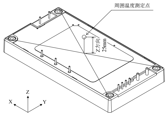
図 7-2 周囲温度測定点
