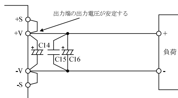
図 6-3 リモートセンシングしない場合 (ローカルセンシング)
