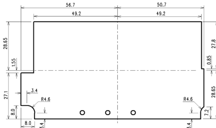
図 7-5 電源カバー外形寸法図
