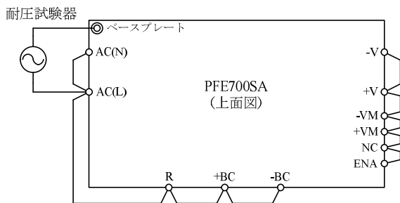
図 6-5 入力-ベースプレート間耐電圧試験方法
