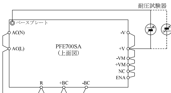
図 6-5 入力-ベースプレート間耐電圧試験方法
