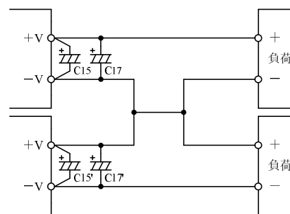
図 6-3 正出力使用の直列運転
