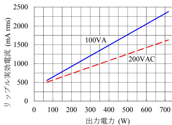
図 5-2 許容リプル電流値
