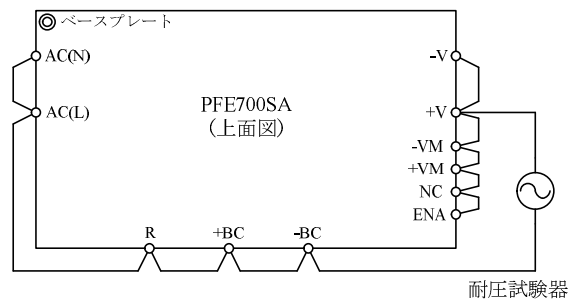
図 6-6 入力-出力間耐電圧試験方法
