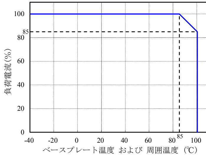
図 7-3 ディレーティングカーブ (負荷電流 対 ベースプレート温度および周囲温度)
