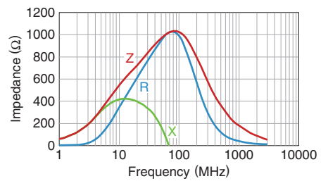
KMZ1608RHR102ATD25
