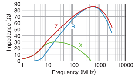
KMZ1608RHR600ATD25
