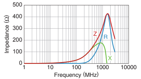
MMZ0603D800CTD25
