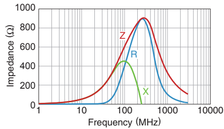
MMZ0603D560CTD25
