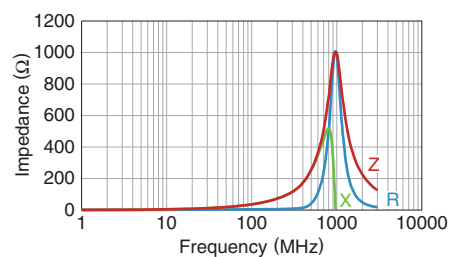
MMZ0603F330CTD25
