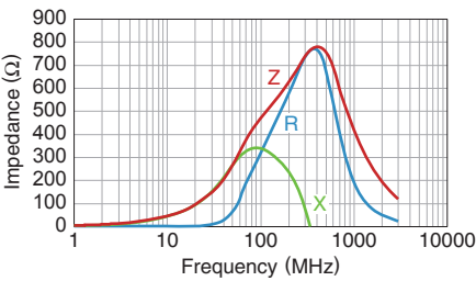
MMZ0603D470CTD25
