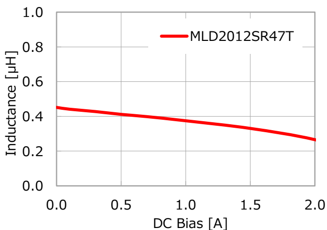
Inductance vs. DC bias (2012055サイズ)
