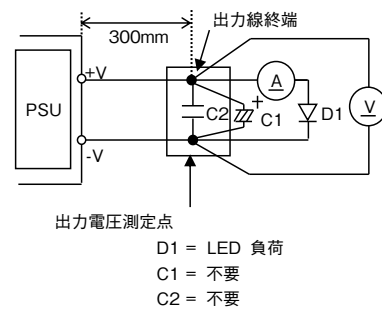
測定回路図
