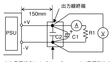
測定回路図
