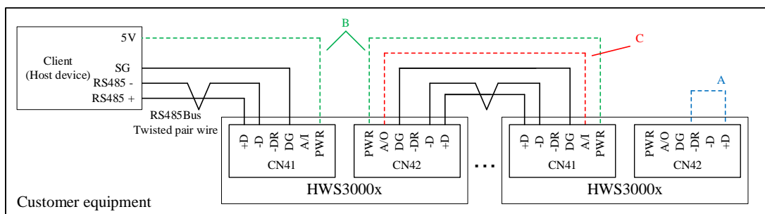
Figure 3-2 Actual wiring
