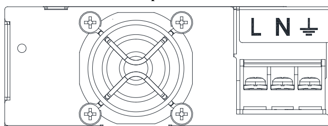
Input side
