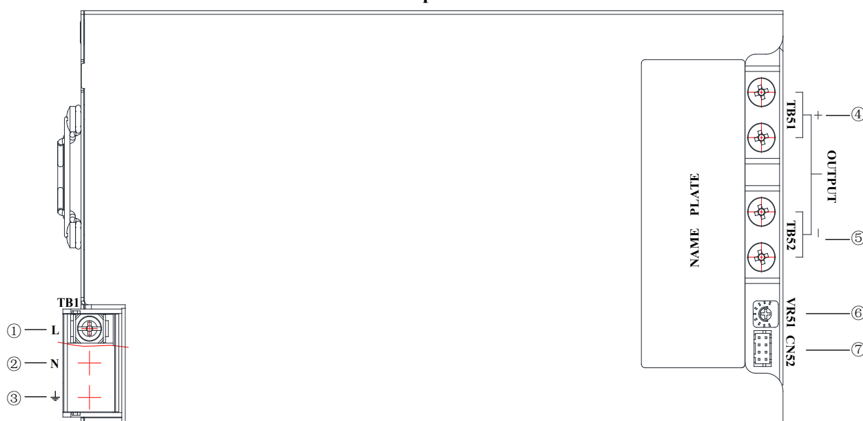
Top side
