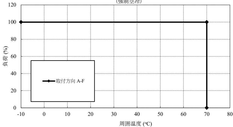
負荷 対 周囲温度 (強制空冷)
