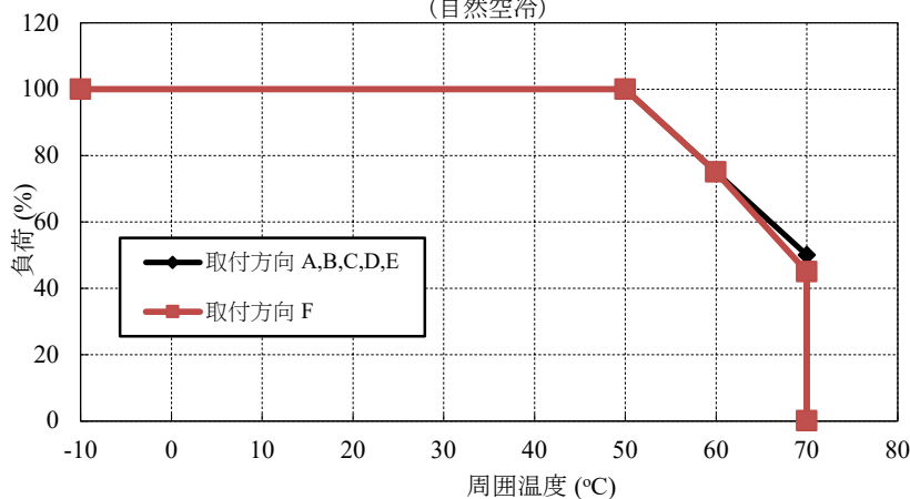
負荷 対 周囲温度 (自然空冷)
