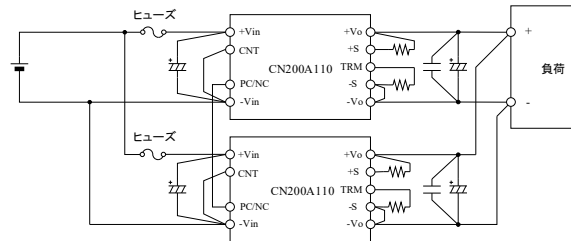
図 12-2 出力電圧可変
