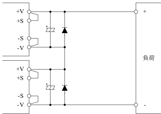
図 13-1 出力電圧積み重ね直列運転
