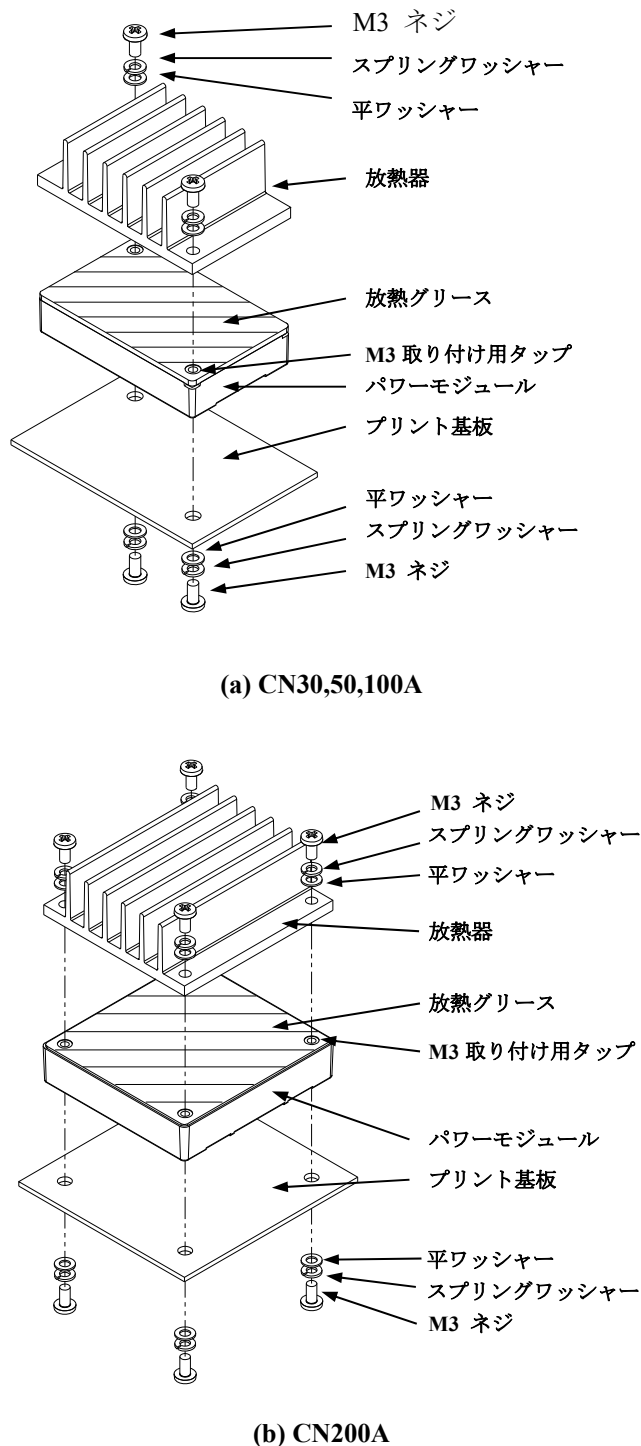
図 1-1 実装方法
