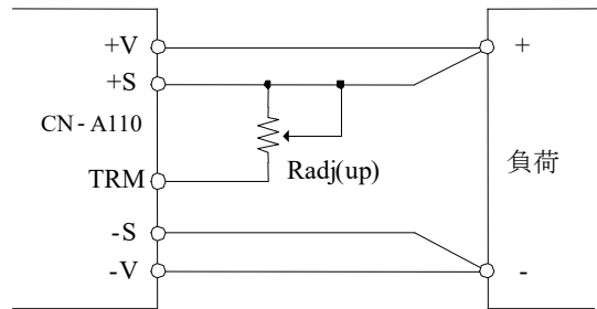
図 2-3 可変抵抗接続(2)
