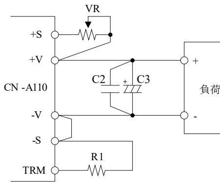
図 2-5 外付け抵抗の接続例
