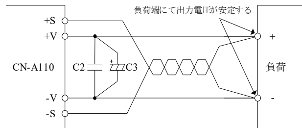
図 10-1 リモートセンシングする場合
