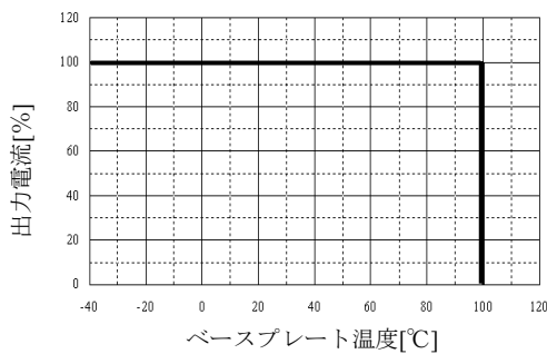
図 15-2 ディレーティングカーブ
