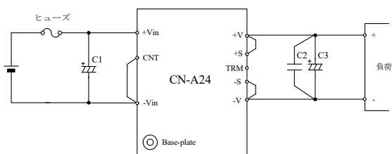
図 1-2 基本的な接続
