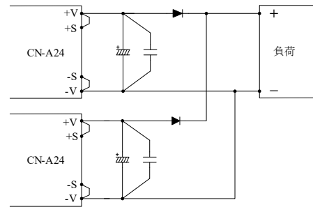
図 12-1 冗長運転接続方法
