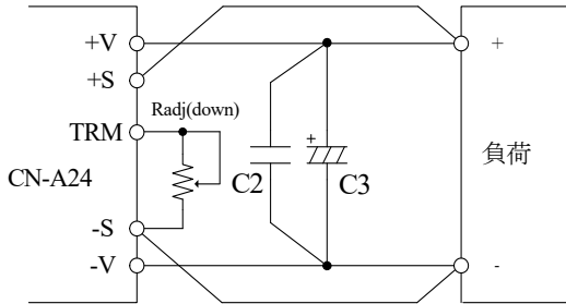
図 2-1 可変抵抗接続(1)
