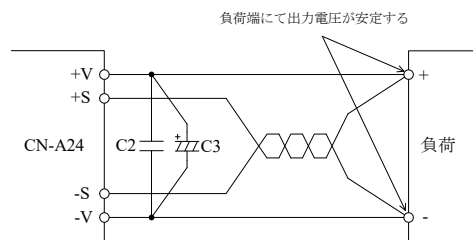
図 10-1 リモートセンシングする場合
