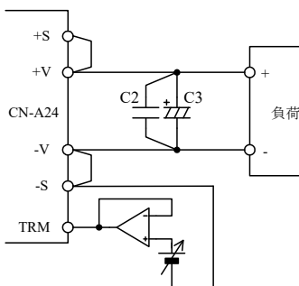
図 2-6 外部電圧印加の接続例
