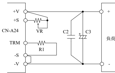
図 2-5 外付け抵抗の接続例
