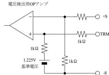
図 2-7 トリム回路構成 (参考)
