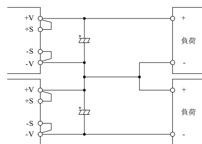
図 14-2 ±出力使用の直列運転
