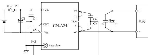
図 20-4 外付け部品接続例
