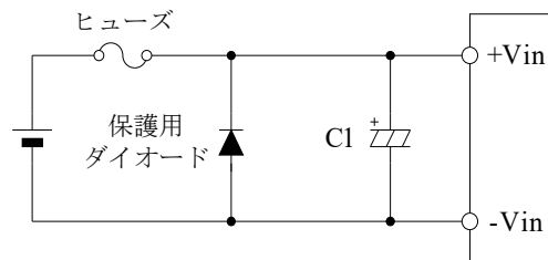
図 1-3 入力の逆接続保護
