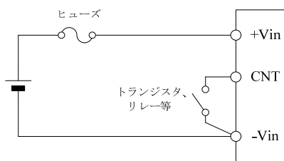
図 11-1 CNT 接続例 (1)
