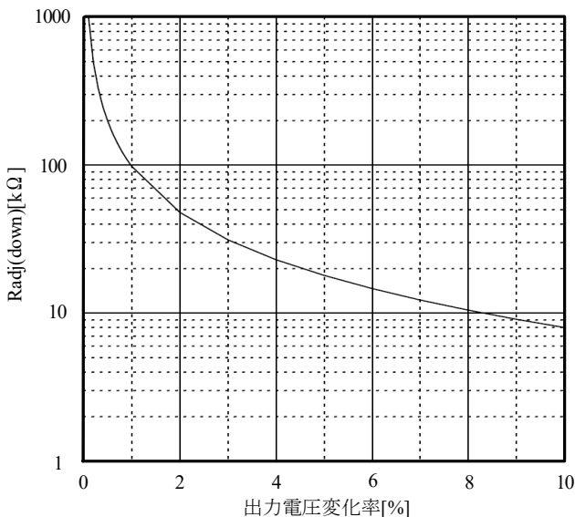
図 2-2 Δ(%)對外付け抵抗(1)
