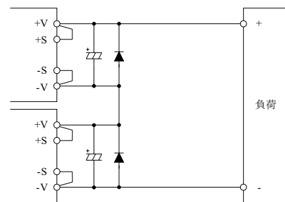
図 14-1 出力電圧積み重ね直列運転
