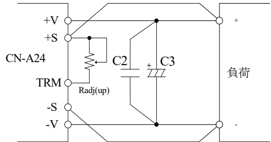
図 2-3 可変抵抗接続(2)
