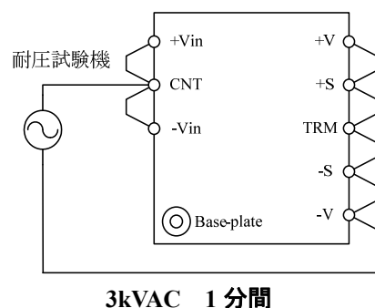
図 20-1 入力-出力間耐電圧試験方法
