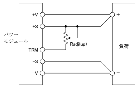
図 2-4 可変抵抗接続(2)
