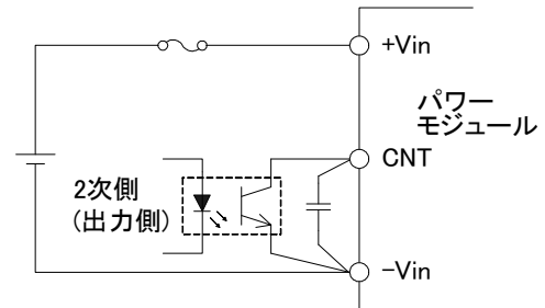
図 10-2 CNT 接続例 (2)
