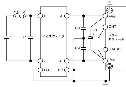
図 1-6 EMI 対策用推奨入力フィルタ (1)
