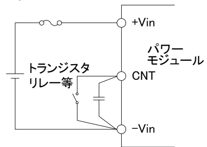
図 10-1 CNT 接続例 (1)
