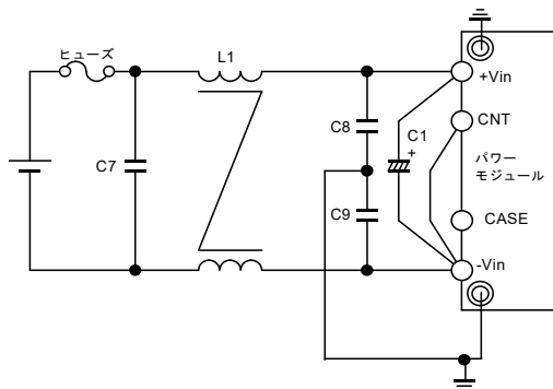
図 1-7 EMI 対策用推奨入力フィルタ (2)
