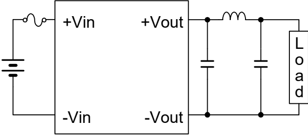
図8 出力リップルノイズを低減する接続 Fig8 Connection to reduce output ripple Voltage
