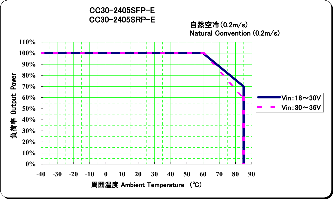
図 2-3 パワーディレーティング (CC30-2405SxP-E) Fig2-3 Power Derating (CC30-2405SxP-E)
