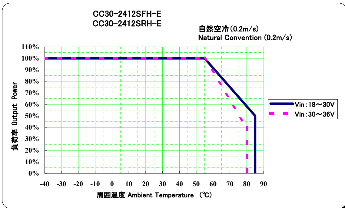
図 2-8 パワーディレーティング (CC30-2412SxH-E) Fig2-8 Power Derating (CC30-2412SxH-E)
