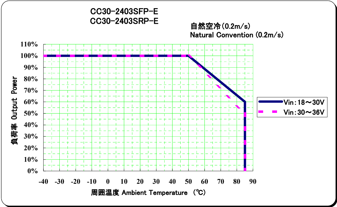
図 2-2 パワーディレーティング (CC30-2403SxP-E) Fig2-2 Power Derating (CC30-2403SxP-E)
