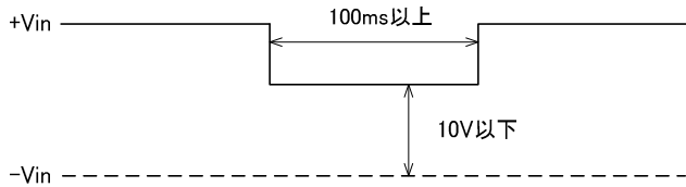
図5 リセット条件 (Vin) Fig5 Reset condition (Vin)
