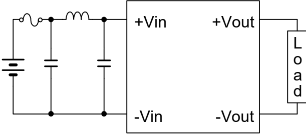
図7 入力帰還ノイズを低減する接続 Fig7 Connection to reduce input feedback Noise
