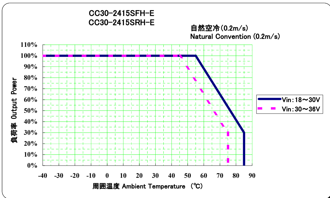
図 2-9 パワーディレーティング (CC30-2415SxH-E) Fig2-9 Power Derating (CC30-2415SxH-E)
