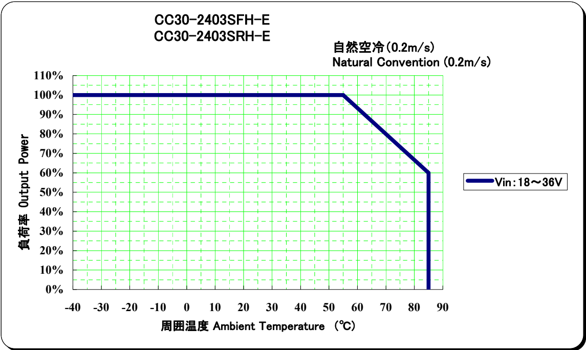
図 2-6 パワーディレーティング (CC30-2403SxH-E) Fig2-6 Power Derating (CC30-2403SxH-E)
