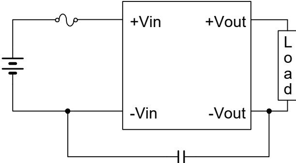
図9 コモンモードノイズを低減する接続 Fig9 Connection to reduce common mode noise
