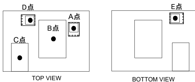
図 2-1 測定ポイント
