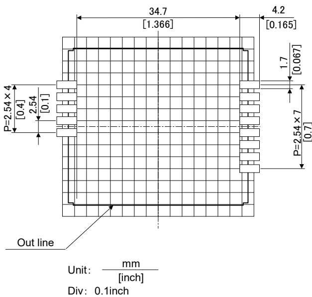
図 13 SMD タイプ推奨基板パッドデザイン (上面図)
