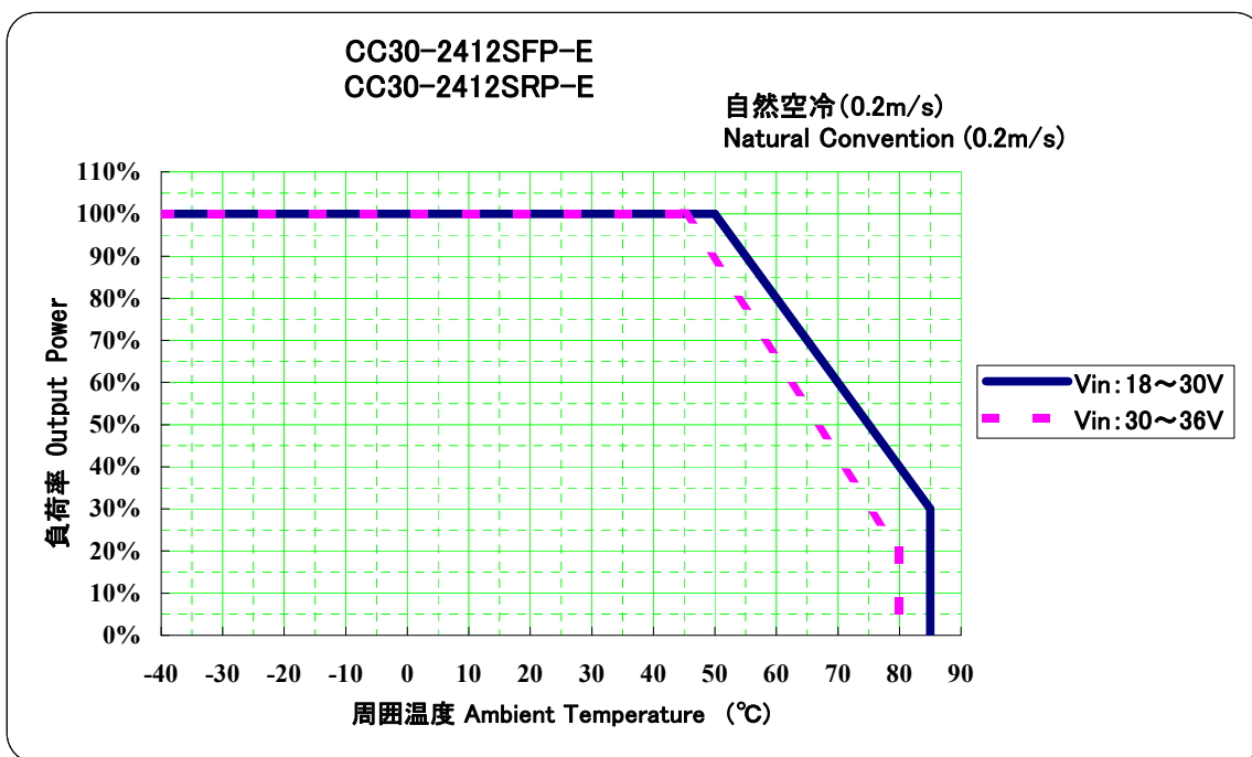
図 2-4 パワーディレーティング (CC30-2412SxP-E) Fig2-4 Power Derating (CC30-2412SxP-E)
