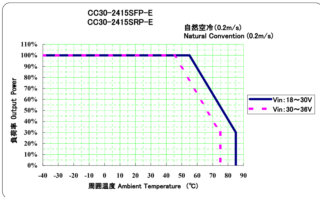
図 2-5 パワーディレーティング (CC30-2415SxP-E) Fig2-5 Power Derating (CC30-2415SxP-E)
