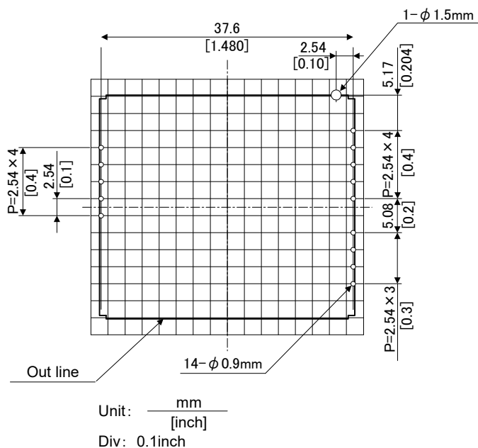
図 12 DIP タイプ推奨基板パッドデザイン (上面図)
