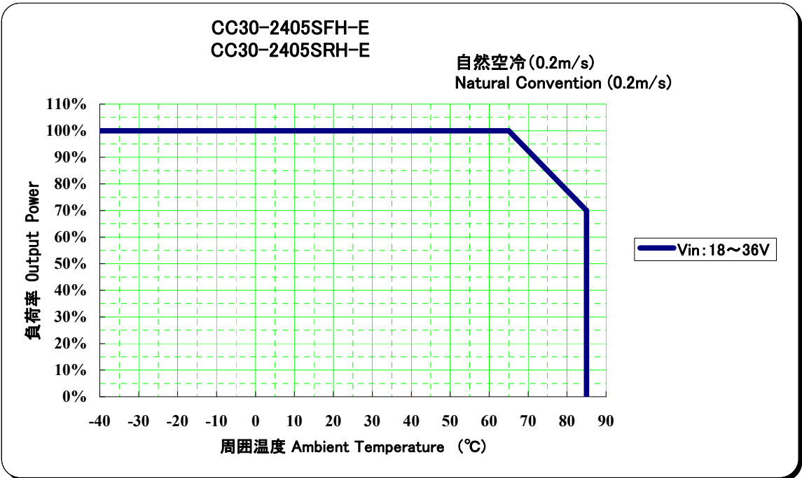
図 2-7 パワーディレーティング (CC30-2405SxH-E) Fig2-7 Power Derating (CC30-2405SxH-E)
