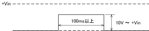
図6 リセット条件 (Vrc) Fig6 Reset condition (Vrc)
