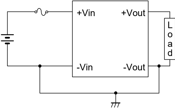
図10 非絶縁で使用する場合の接続 Fig10 Connection to use non-isolation
