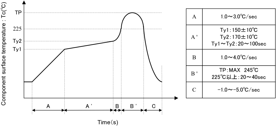
図4 SMDタイプのリフロープロセス条件 Fig4 Reflow process conditions for SMD type.
