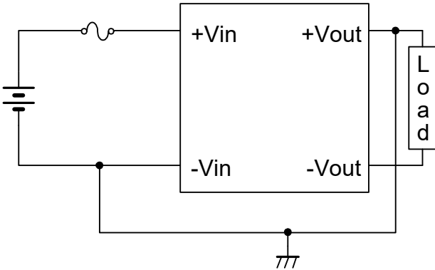
図11 極性反転出力(非絶縁)で使用する場合の接続 Fig11 Connection to use turn around output voltage (non-isolation)
