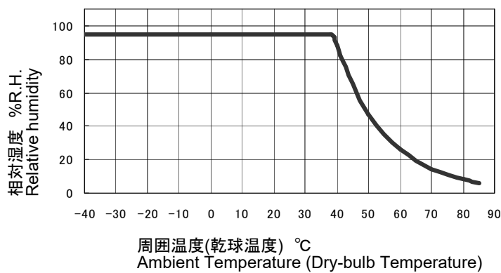
図1 湿度ディレーティング
