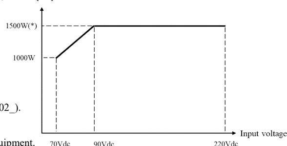
Fig.B Output power
