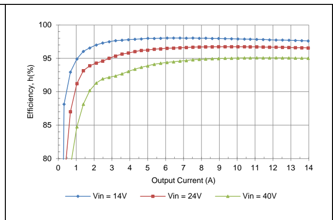
V_o = 12\text{ V}
