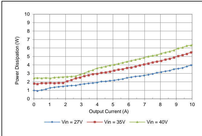
Vo = 24 V
