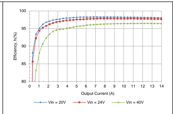
V_o = 18\text{ V}
