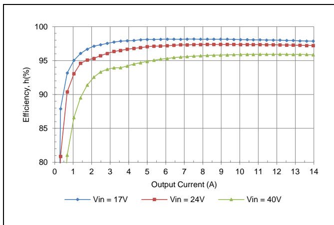
V_o = 15\text{ V}
