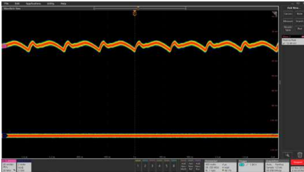
Vo ripple 12.5 mV @ 0 A Ch7: Vo CH6: Io
