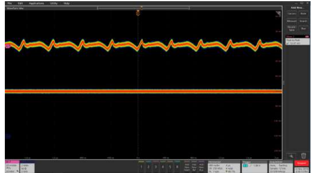
Vo ripple 12.4 mV @ 6 A Ch7: Vo CH6: Io
