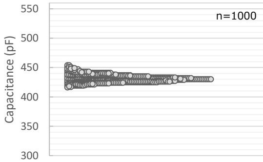
Capacitance Dispersion ※1kHz, 1Vrms
