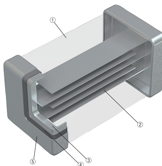
図2 積層チップサーミスタの内部構造
